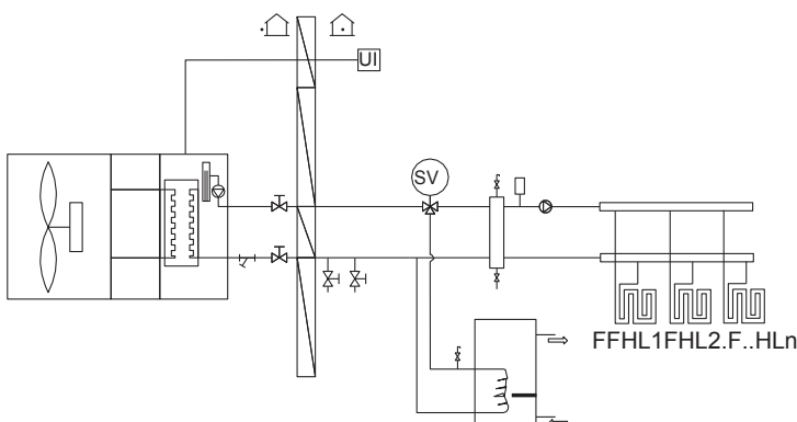
2 sistemos išdėstymas
