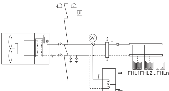
1 sistemos išdėstymas
